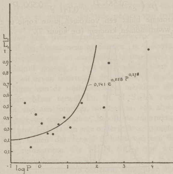
Fig. 6. Toenemende helderheid van den begeleider ten opzichte van de hoofdstel bij toenemende periode.
