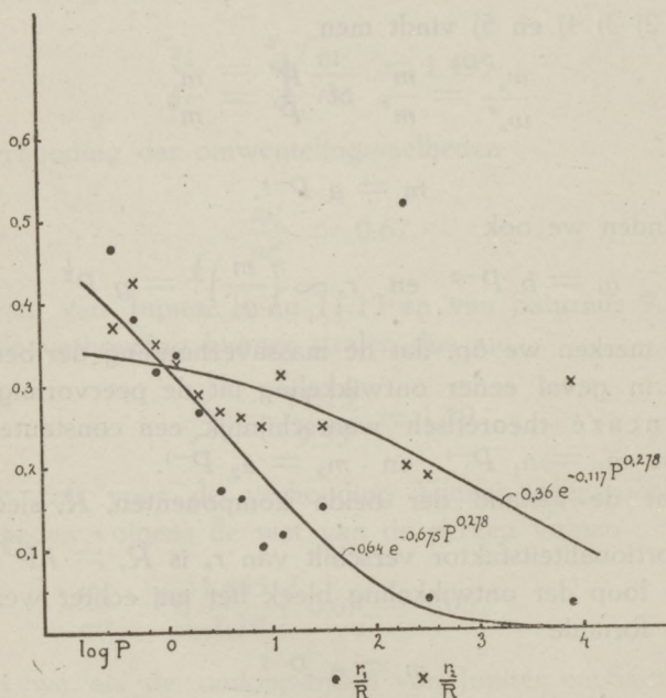
Fig. 4. Een beeld van de afnemende der quotiënten r_1/R en r_2/R met toenemende periode.
