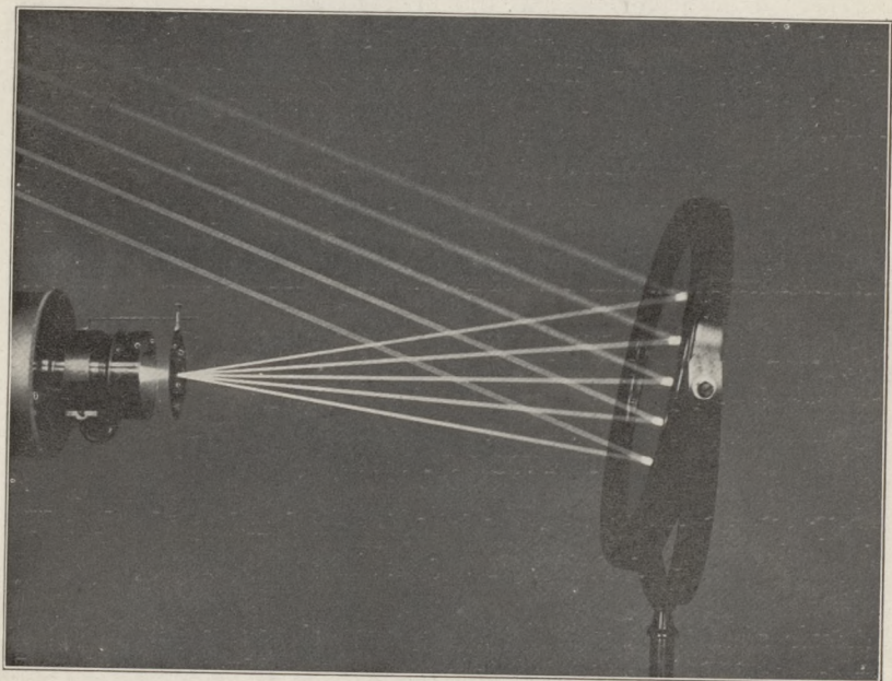
No. 7. Lichtend punt in het hoofdbrandpuntsvlak van een hollen spiegel.
